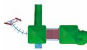
TULA Accesorios plásticos TM002P Capacidad: 20 usuarios Medidas: L: 7.48 m / An: 4.37 m / Al: 3.93 m Área de seguridad: L: 10.18 m / An: 7.07 m
