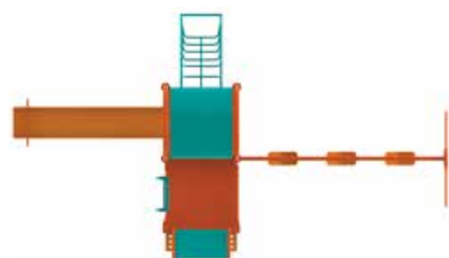
FIESTA TM08B Capacidad: 22 usuarios Medidas: L: 6.24 m / An: 3.95 m / Al: 3.80 m Área de seguridad: L: 8.94 m / An: 6.35 m
