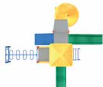
PACHAL NO. 2 TM79P Accesorios Plásticos Capacidad: 26 usuarios Medidas: L: 6.63 m / An: 5.88 m / Al: 3.63 m Área de seguridad: L: 9.33 m / An: 8.88 m
