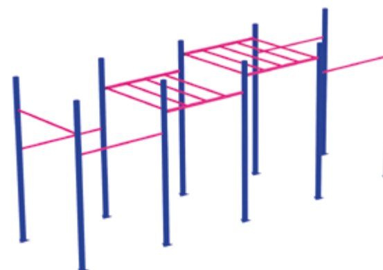
CALISTENIA 07 JIMCAL-07 Capacidad: 7 usuarios L: 6.00 m / An: 1.50 m / Al: 2.50 m
