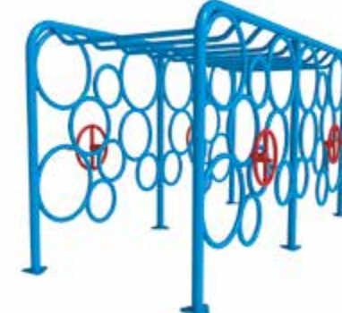
TÚNEL PASAMANOS INC-04 Capacidad: 6 usuarios Medidas: L: 2.90 m / An: 1.60 m / Al: 1.60 m Área de seguridad: L: 6.90 m / An: 5.60 m
