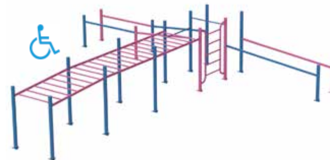
CALISTENIA 15 JIMCAL-15 Capacidad: 9 usuarios L: 8.20 m / An: 8.00 m / Al: 2.00 m
