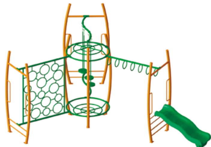
ODYSSEY Accesorios plásticos EXTRE-3 Capacidad: 20 usuarios Medidas: L: 6.50 m / An: 5.62 m / Al: 3.02 m Área de seguridad: L: 9.50 m / An: 8.62 m
