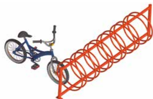
APARCA 02 JIMAB-02 Capacidad: 12 usuarios L: 2.76 m / An: 0.62 m / Al: 0.70 m
