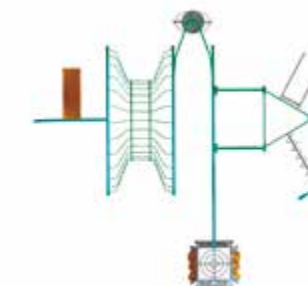
VOLCANO Accesorios plásticos EXTRE-6 Capacidad: 40 usuarios Medidas: L: 9.73 m / An: 8.82 m / Al: 3.00 m Área de seguridad: L: 12.73 m / An: 11.82 m
