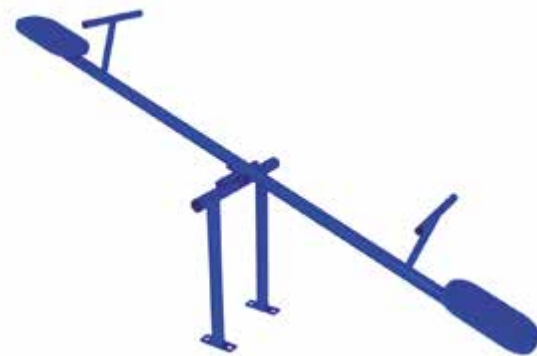
SUBE Y BAJA SENCILLO SYB01 Capacidad: 2 usuarios Medidas: L: 2.32 m / An: 0.50 m / Al: 1.05 m
