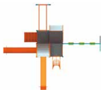
MULTITORRE TM02B Capacidad: 33 usuarios Medidas: L: 8.34 m / An: 7.45 m / Al: 4.16 m Área de seguridad: L: 11.04 m / An: 10.15 m
