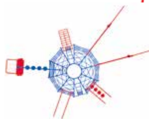
SKY EXTRE-2 Capacidad: 45 usuarios Medidas: L: 10.34 m / An: 7.99 m / Al: 2.91 m Área de seguridad: L: 13.34 m / An: 10.99 m
