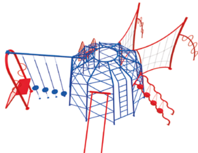
SKY EXTRE-2 Capacidad: 45 usuarios Medidas: L: 10.34 m / An: 7.99 m / Al: 2.91 m Área de seguridad: L: 13.34 m / An: 10.99 m
