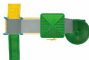
MARCELL Accesorios plásticos TM023P Capacidad: 20 usuarios Medidas: L: 5.62 m / An: 3.86 m / Al: 4.08 m Área de seguridad: L: 8.32 m / An: 6.56 m
