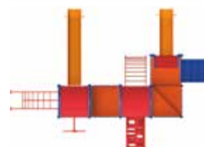
VIENA TM06B Capacidad: 34 usuarios Medidas: L: 6.83 m / An: 5.18 m / Al: 4.17 m Área de seguridad: L: 9.23 m / An: 7.88 m
