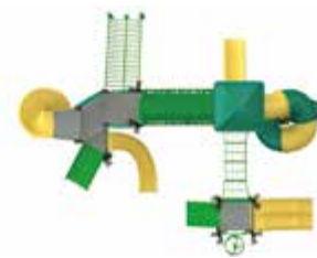
BOSQUES 03 TM87P Accesorios plásticos Capacidad: 60 usuarios Medidas: L: 9.84 m / An: 7.95 m / Al: 5.60 m
