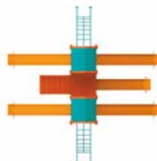
UP-DOWN TM09B Capacidad: 28 usuarios Medidas: L: 6.42 m / An: 5.16 m / Al: 4.06 m Área de seguridad: L: 9.42 m / An: 5.56 m
