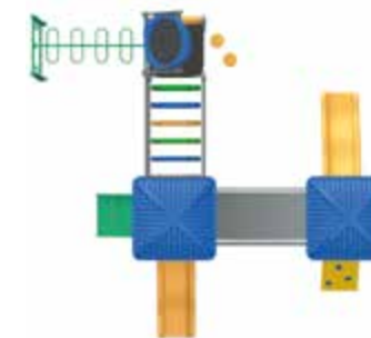
PACHAL NO. 4 Accesorios plásticos TM81P Capacidad: 30 usuarios Medidas: L: 6.05 m / An: 6.55 m / Al: 4.19 m Área de seguridad: L: 8.75 m / An: 8.95 m
