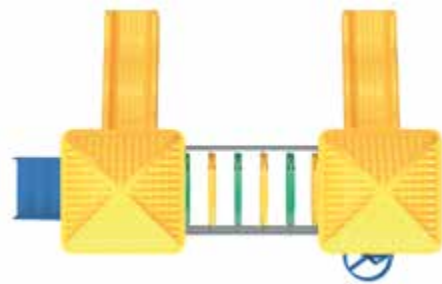
PACHAL NO. 1 Accesorios plásticos TM78P Capacidad: 18 usuarios Medidas: L: 3.55 m / An: 5.39 m / Al: 3.33 m Área de seguridad: L: 5.95 m / An: 8.09 m
