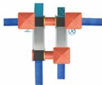
PACHAL NO. 7 Accesorios plásticos TM84P Capacidad: 46 usuarios Medidas: L: 7.86 m / An: 9.43 m / Al: 3.63 m Área de seguridad: L: 10.56 m / An: 12.43 m
