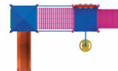
KANT Accesorios plásticos TM77P Capacidad: 16 usuarios Medidas: L: 4.50 m / An: 2.85 m / Al: 3.10 m Área de seguridad: L: 6.90 m / An: 5.55 m
